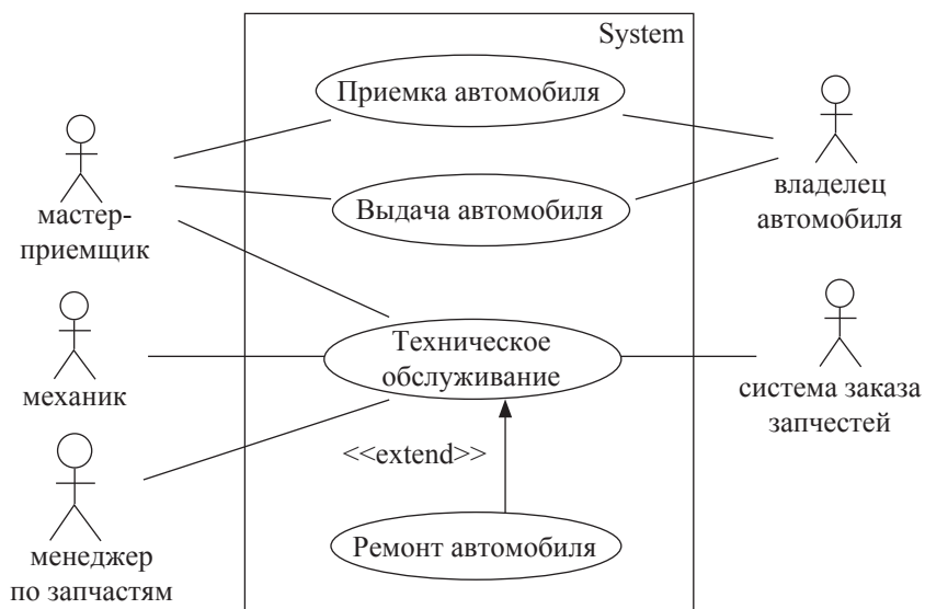
Рис. 5.8. Пример диаграммы прецедентов
